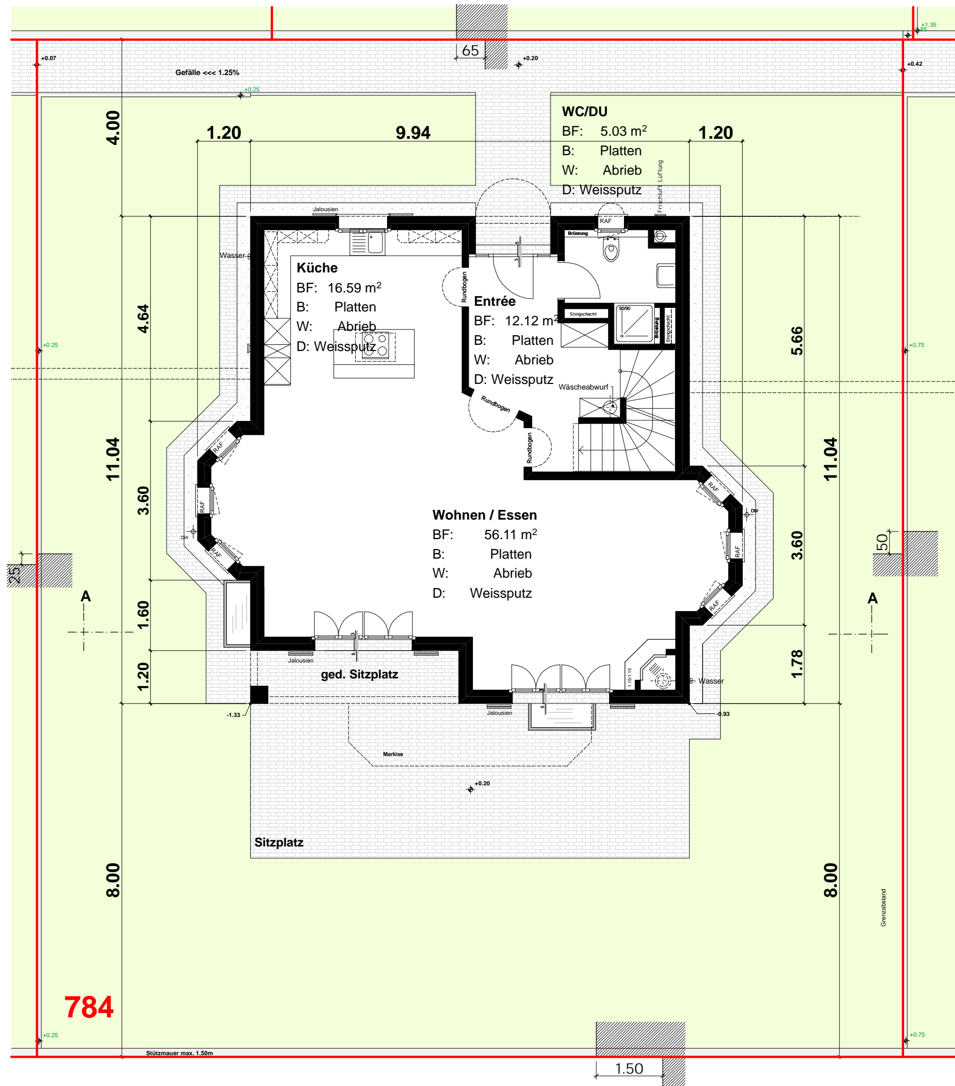
Grundriss EFH Haustyp F Erdgeschoss
